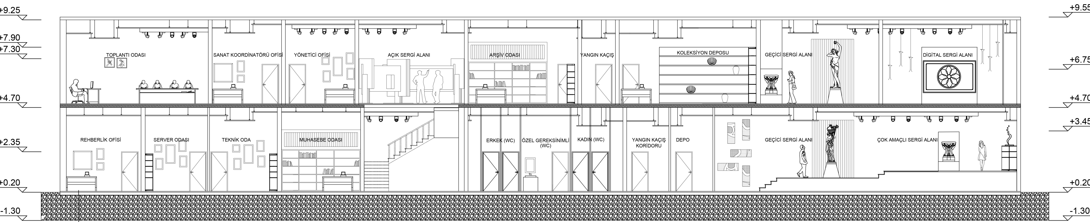
A-A KESİT Ö:1/100
