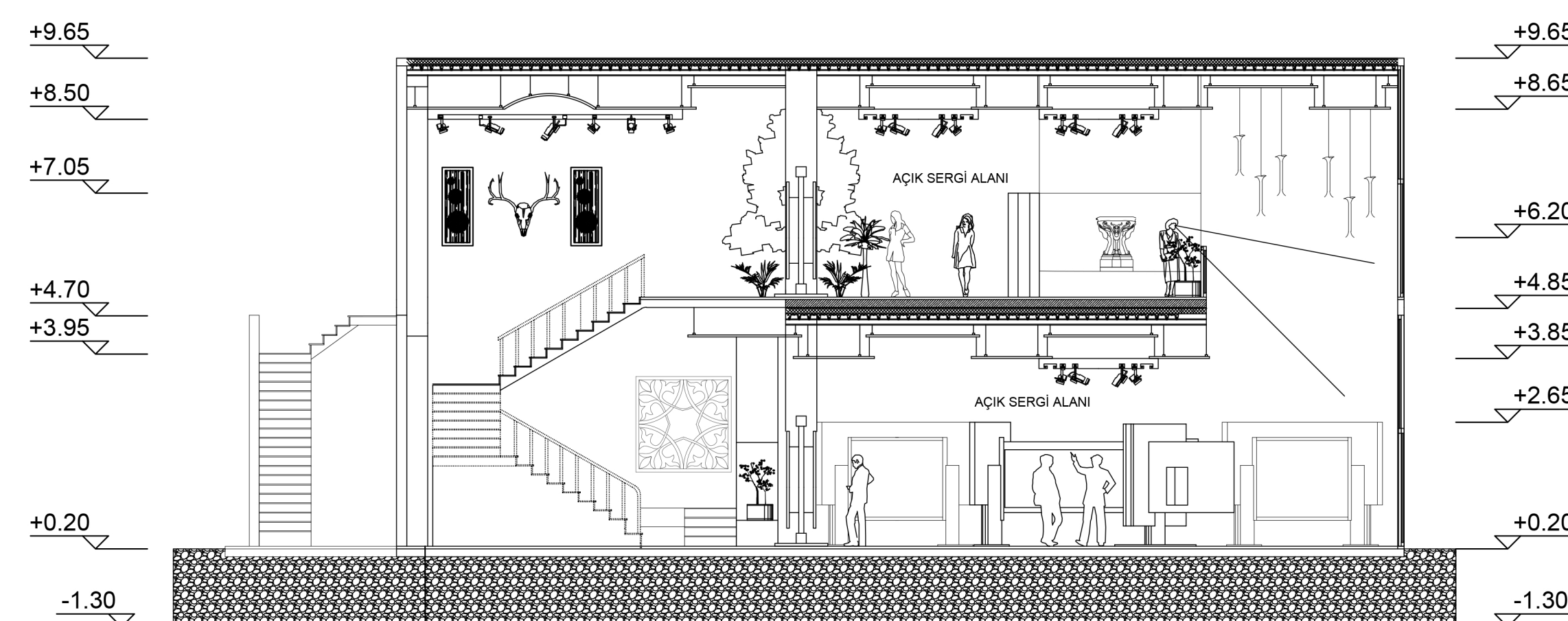
B-B KESİT Ö:1/100
