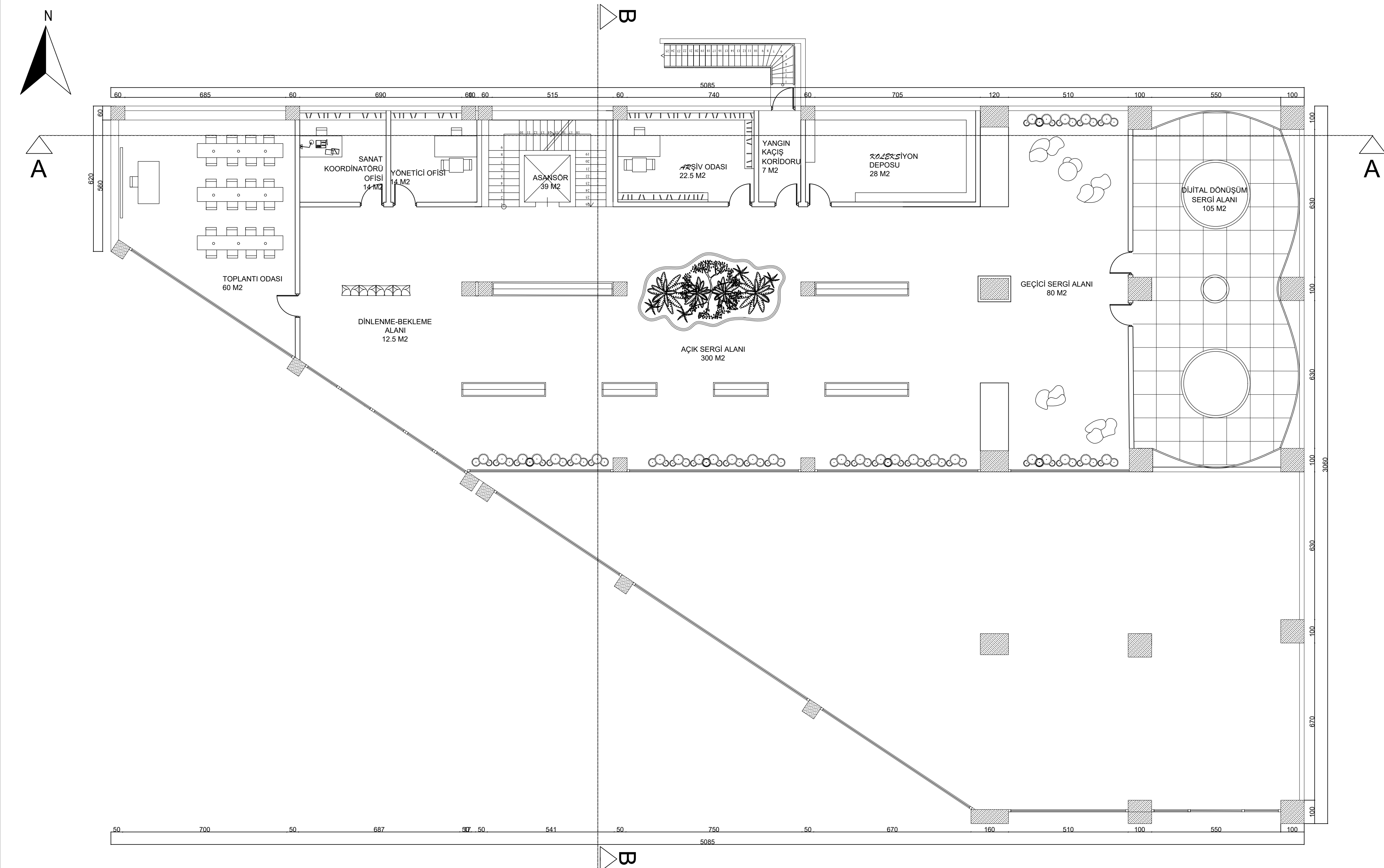
(+4,65) ASMA KAT PLANI Ö:1/100
