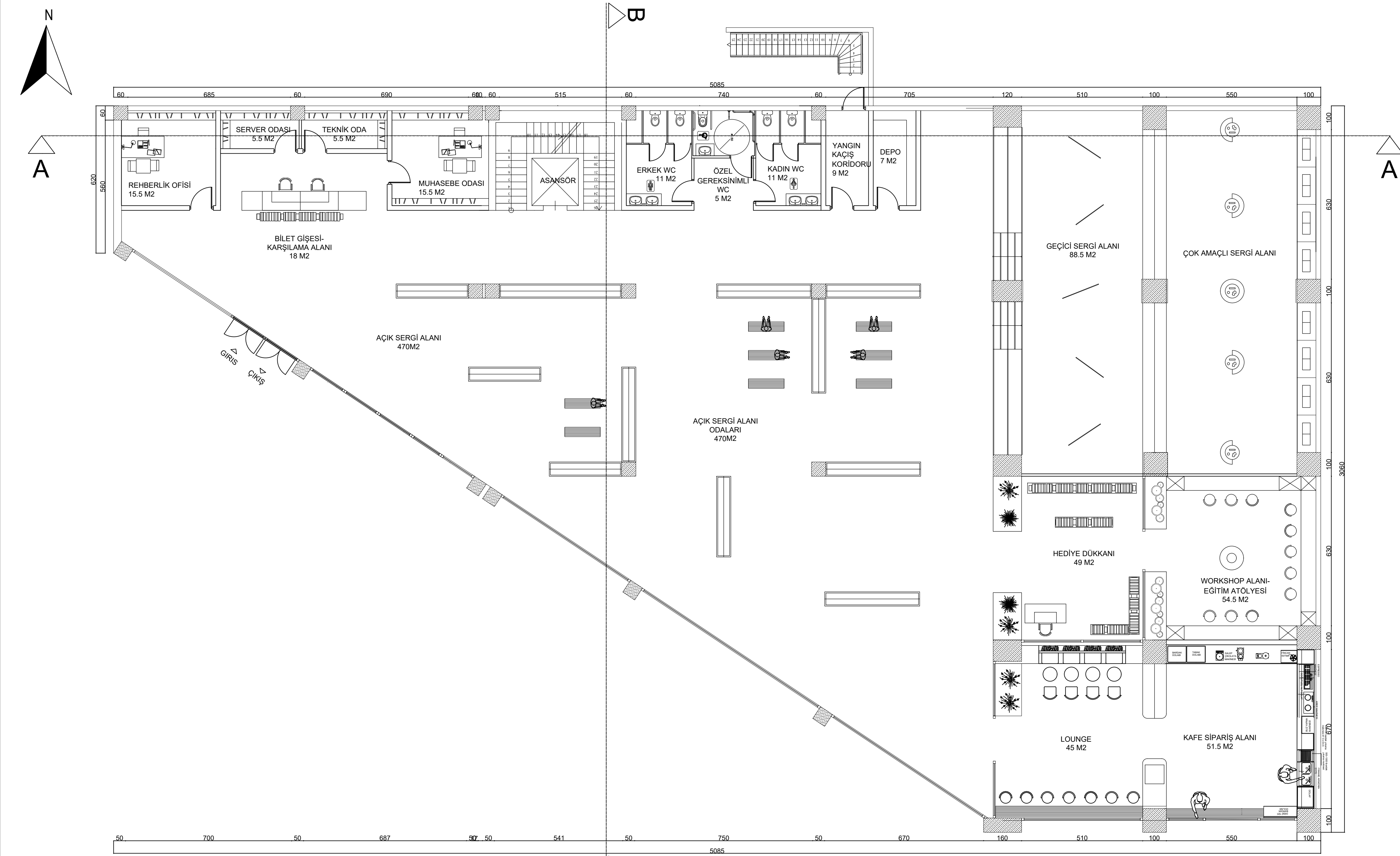
(+0,15) ZEMİN KAT PLANI Ö:1/100
