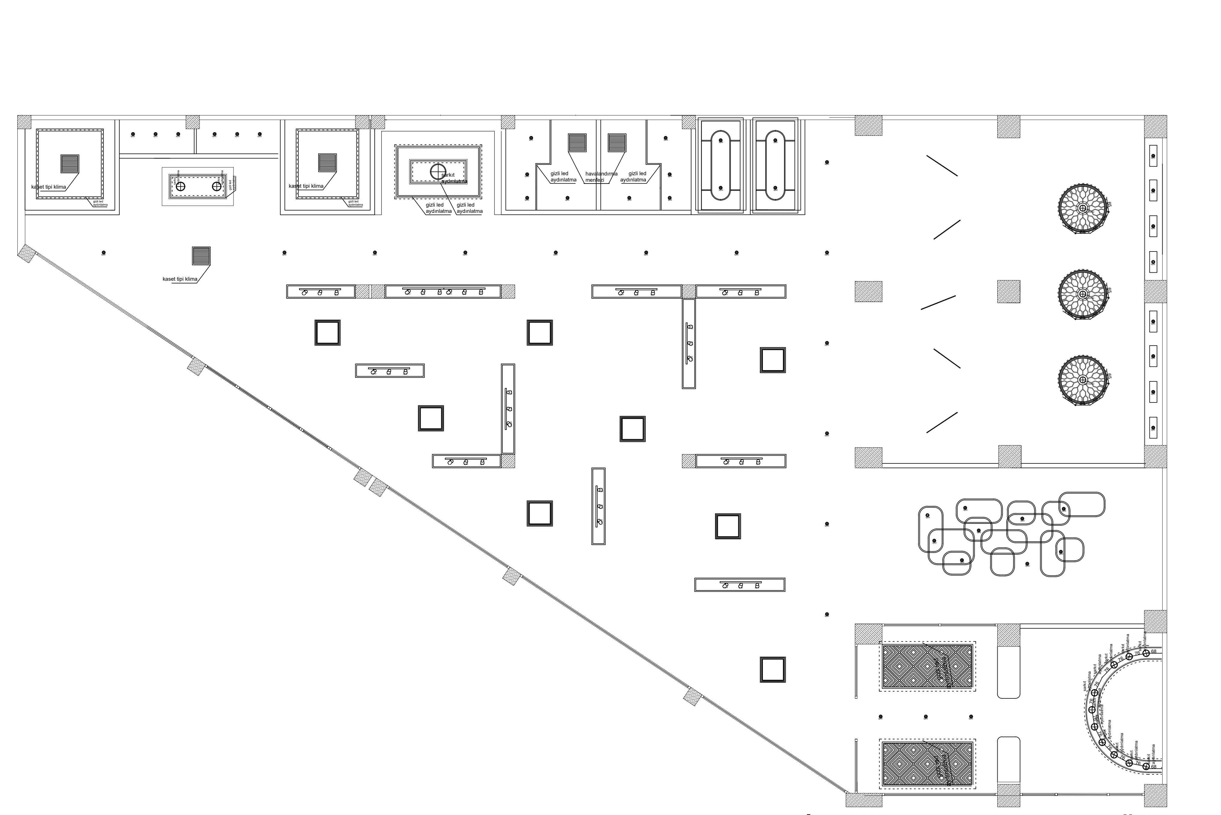
ZEMİN KAT TAVAN PLANI Ö:1/100
