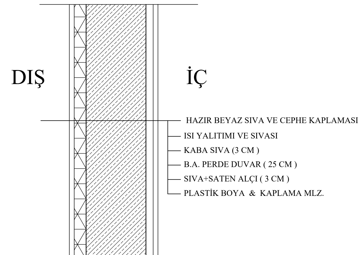
DUVAR DETAYI Ö:1/10
