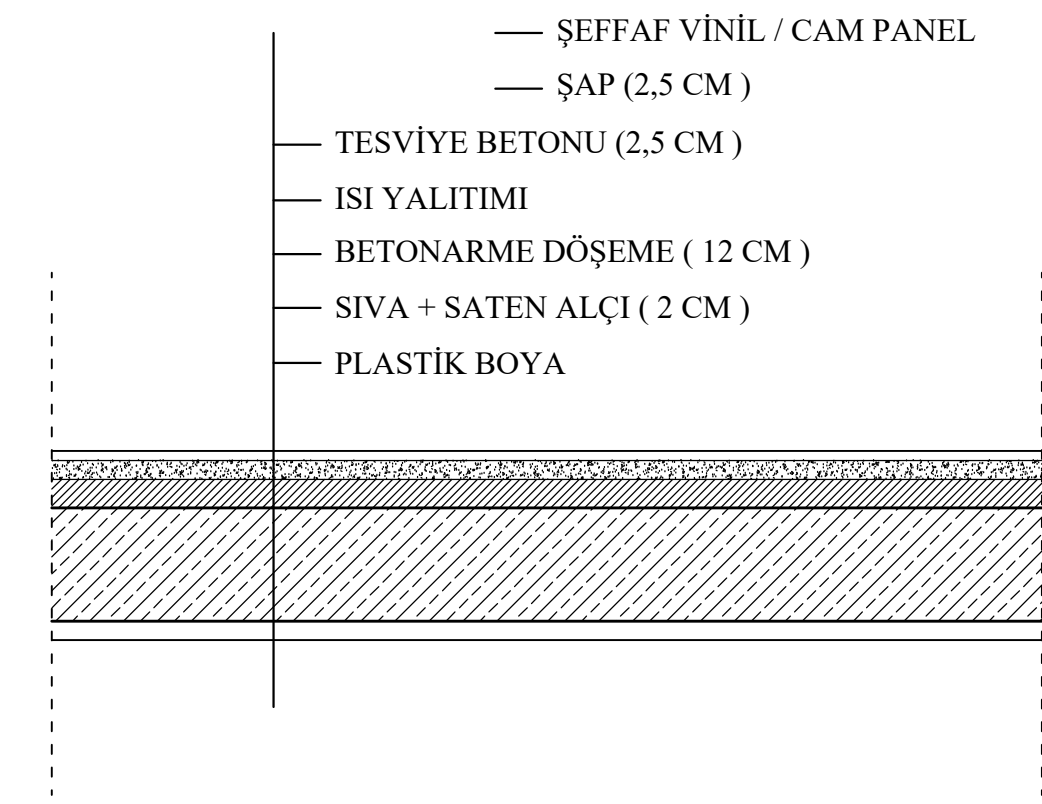
DÖŞEME DETAYI Ö:1/10
