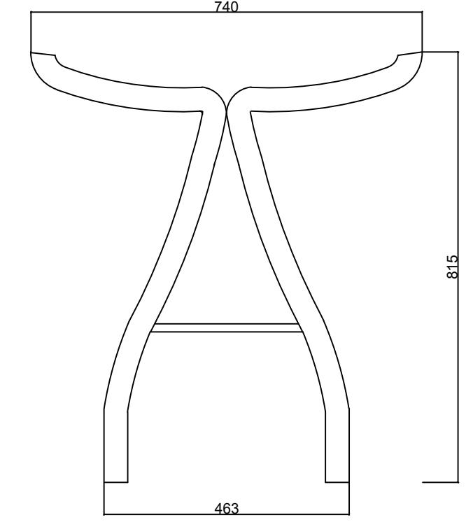
A-A KESİTİ
